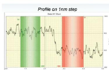
1 nmの膜厚段差測定
